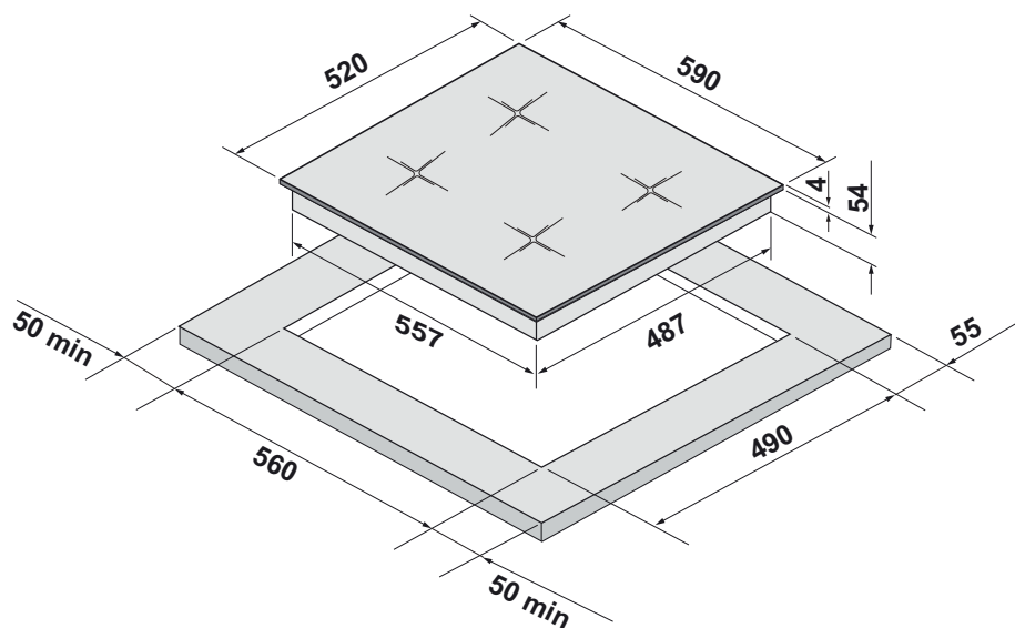
Схема встраивания варочной поверхности
