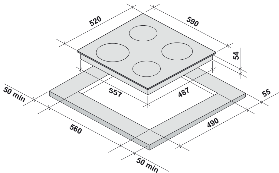
Схема встраивания варочной поверхности КРИН03
